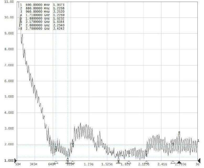
173 S11 SWR 1.000/ Ref 1.000
