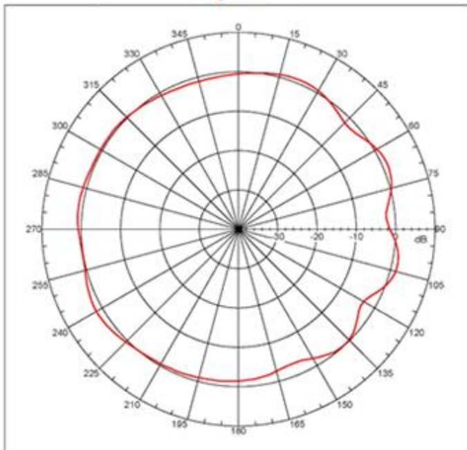
H-plane
