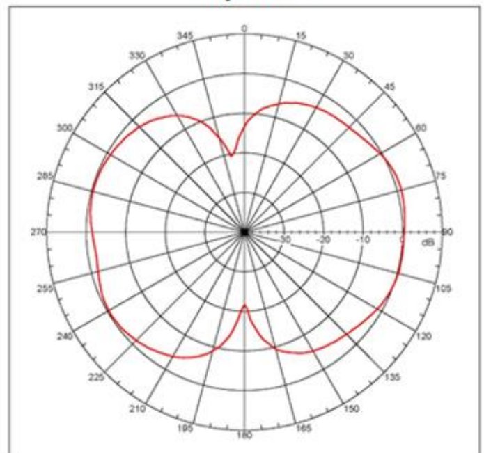
E-plane
