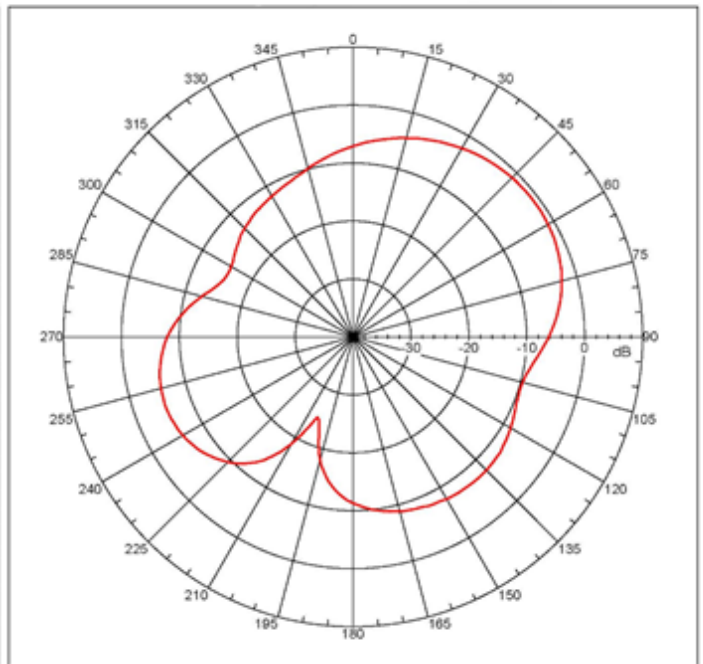
E-plane
