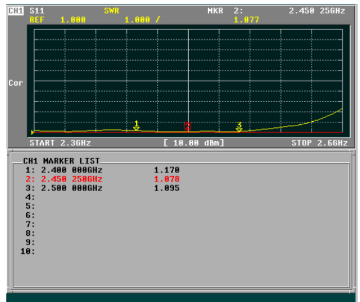
V.S.W.R
