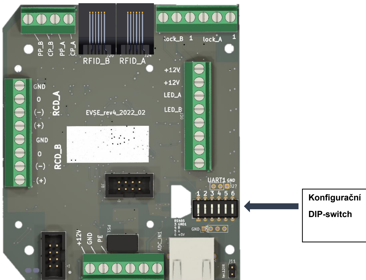
Obrázek 4: Vyznačení DIP-switchu na řídicí desce
