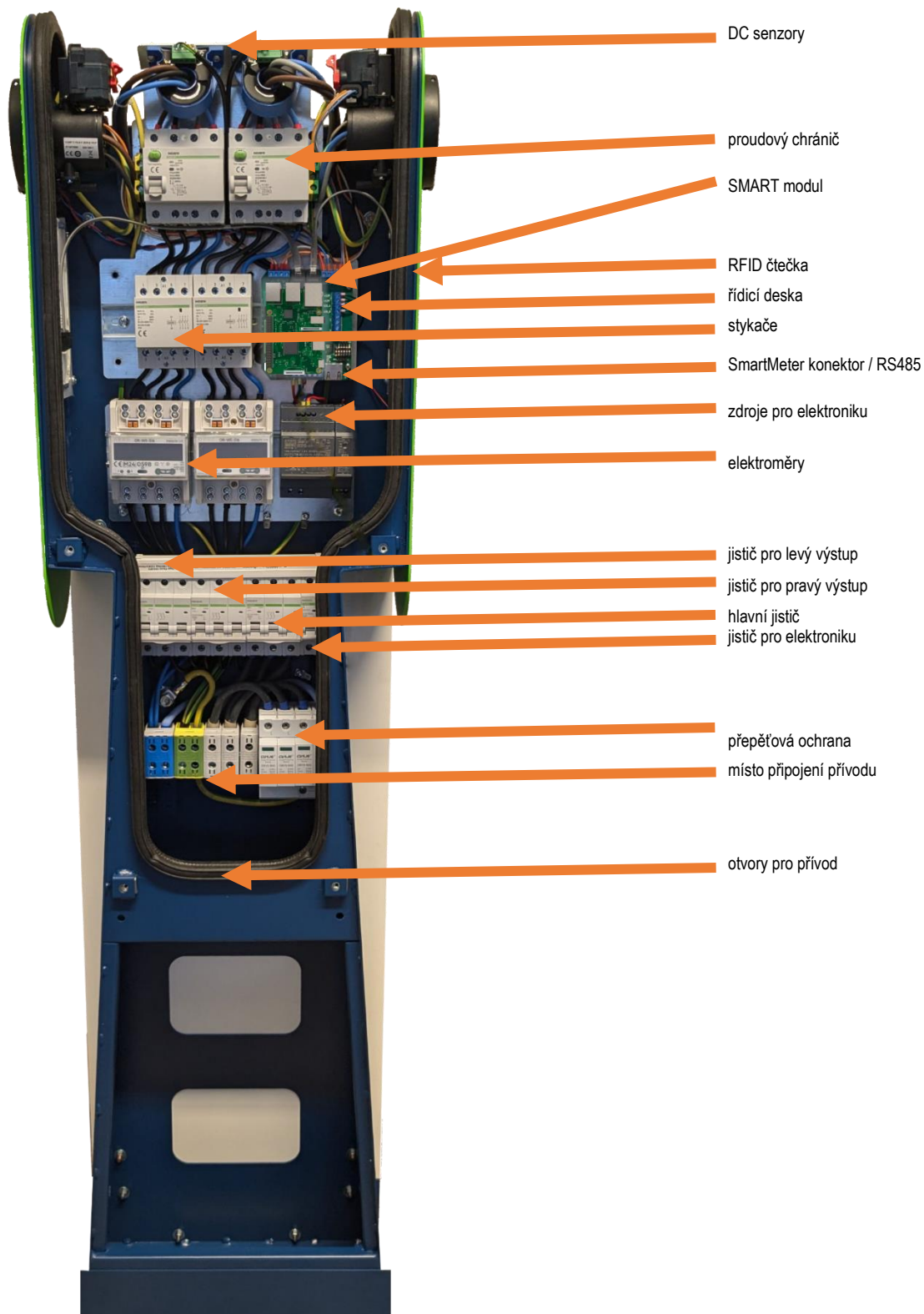
Obrázek 2: přehled komponentů stanice AC lite
