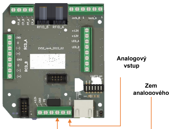
Obrázek 9: Zapojení řídicího vodiče
