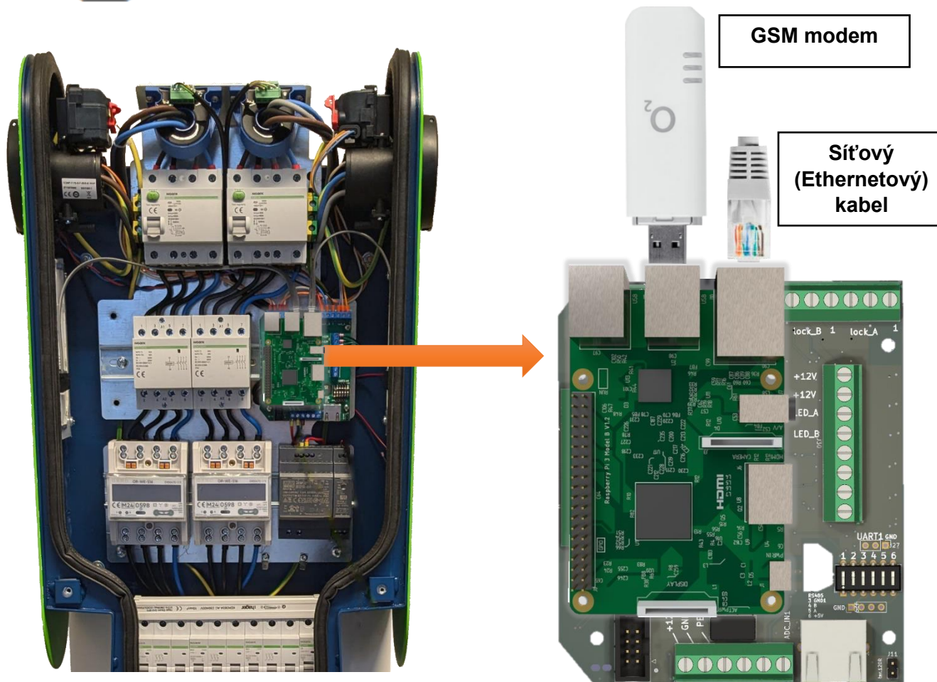
Obrázek 3: Zapojení GSM modemu/síťového kabelu
