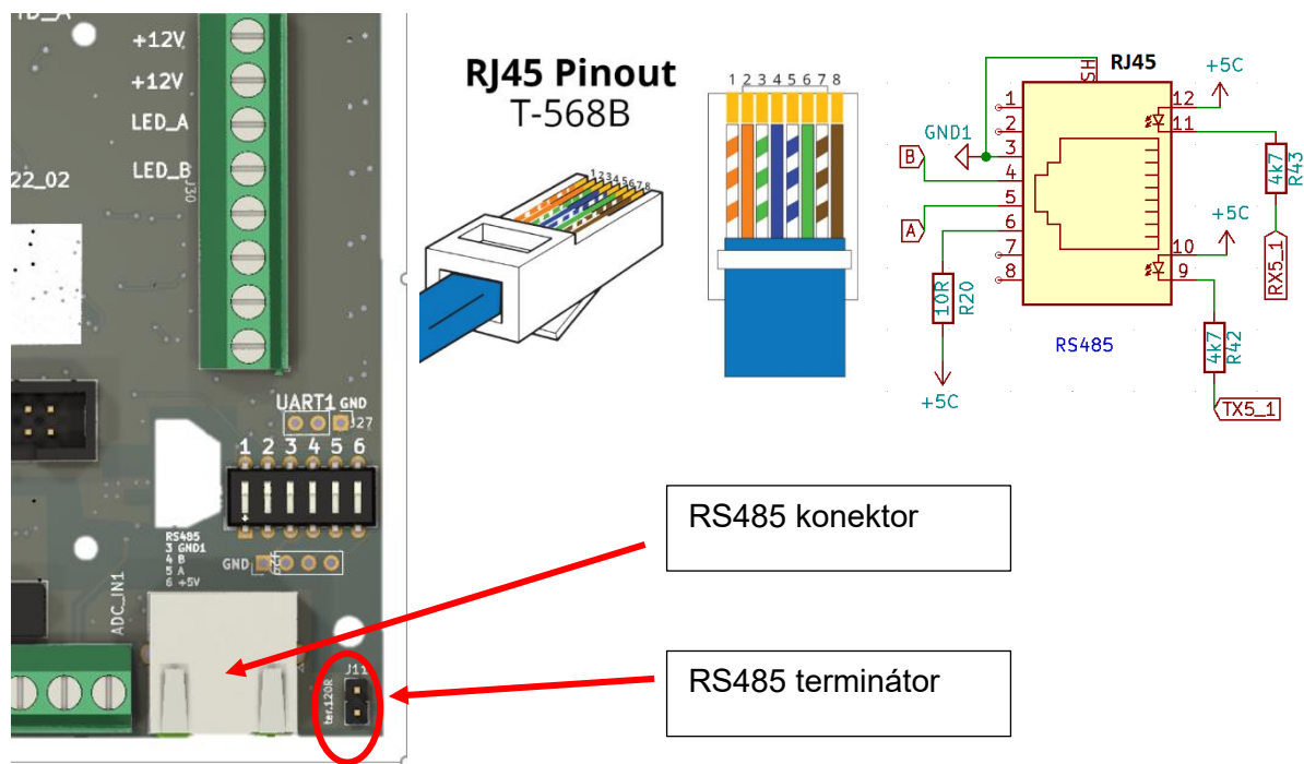
Obrázek 8: RS485 zapojení
