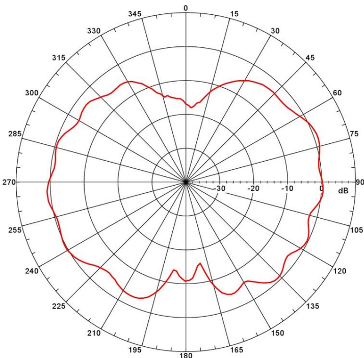
E-PLANE
