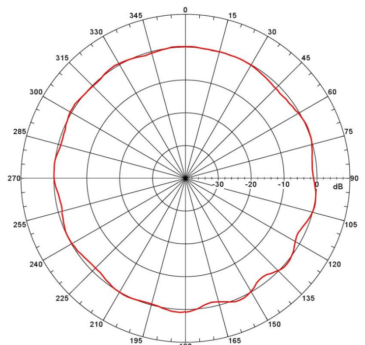
H-PLANE
