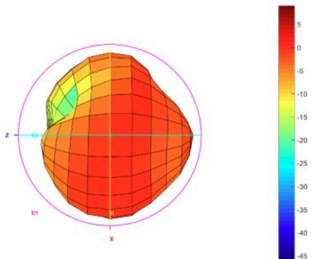
Total_3D_Top View_900MHz
