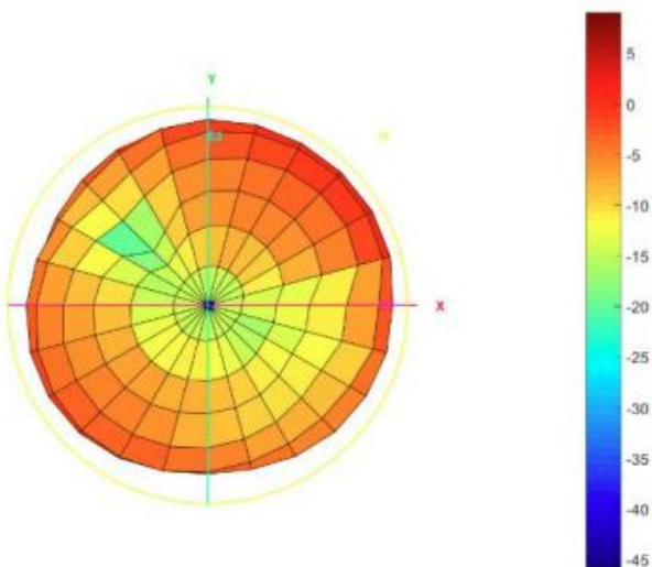
Total_3D_Front View_900MHz
