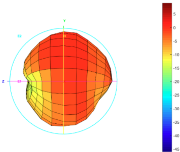
Total_3D_Left View_900MHz
